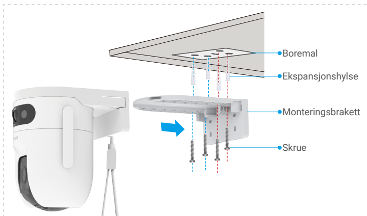
Fig. 1 Takmontering
